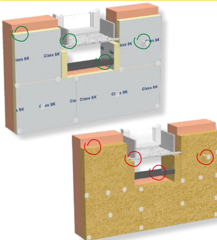
Isolamento a cappotto su pareti in laterizio monostrato da mm 250 Zona Climatica E Trasmittanza Termica richiesta U = 0,28 \text{ W/m}^2\text{K}
